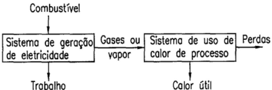
Figura 7: Ciclo topping .
