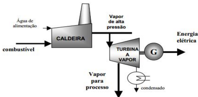
Figura 9: Ciclo Rankine de potência a vapor.
