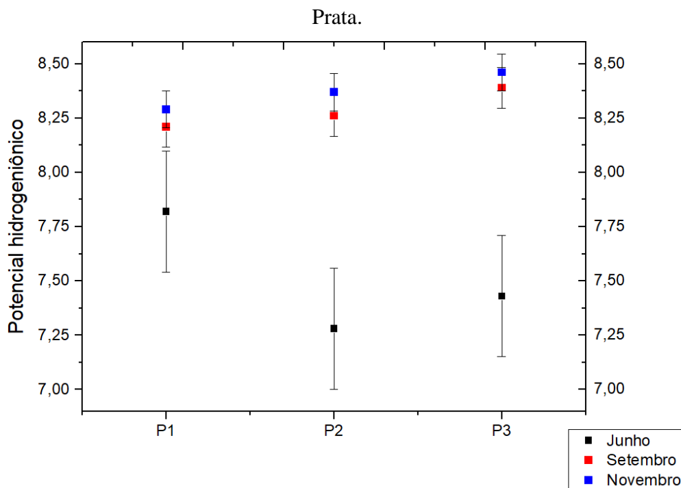
Figura 14 – Variação espacial e sazonal do potencial hidrogeniônico na água do rio da
