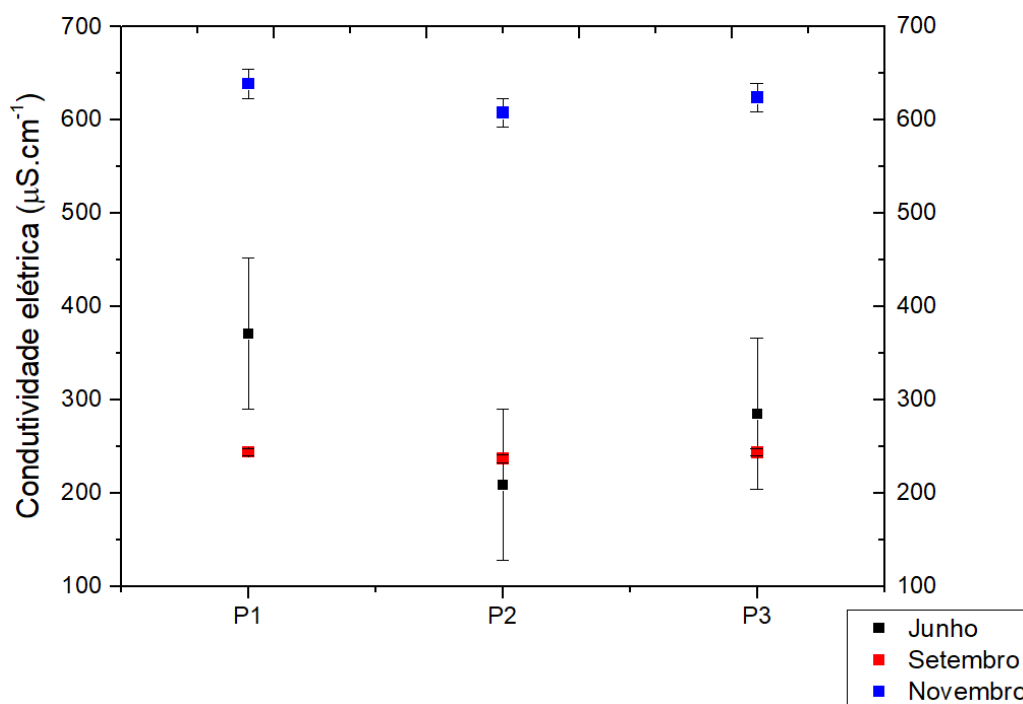
Figura 10 – Variação espacial e sazonal da condutividade elétrica na água do rio da Prata.
