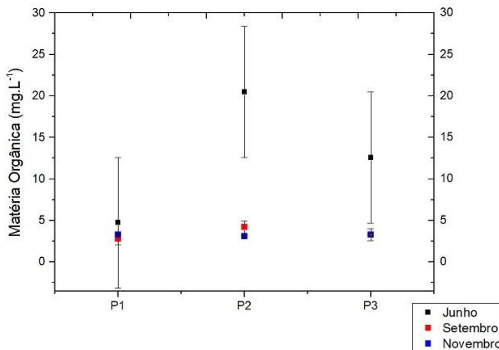
Figura 12 – Variação espacial e sazonal da matéria orgânica na água do rio da Prata.
