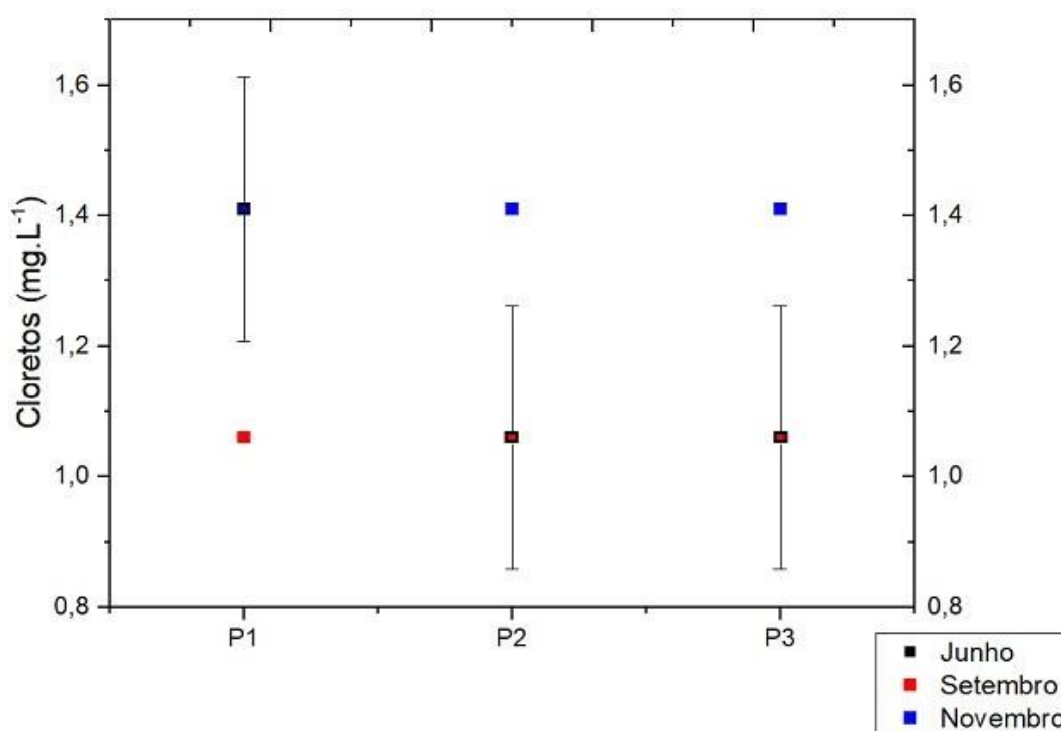
Figura 9 – Variação espacial e sazonal de íons cloretos na água do rio da Prata.
