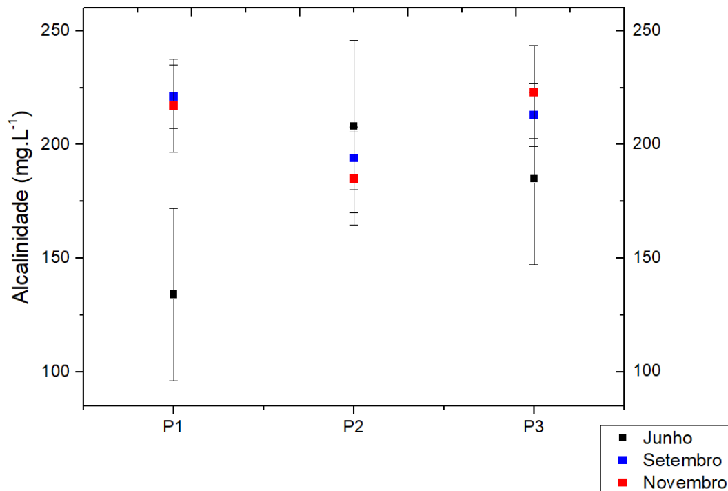
Figura 8 – Variação espacial e sazonal da alcalinidade na água do rio da Prata.
