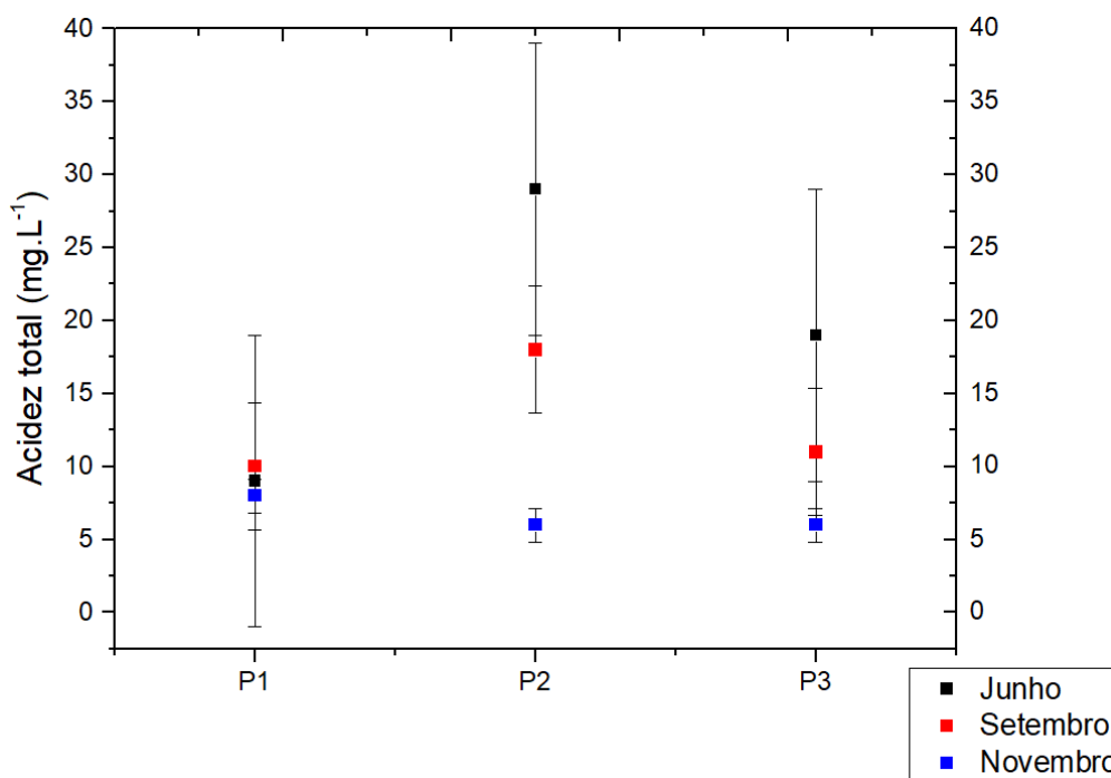
Figura 7 – Variação espacial e sazonal da acidez total na água do rio da Prata.
