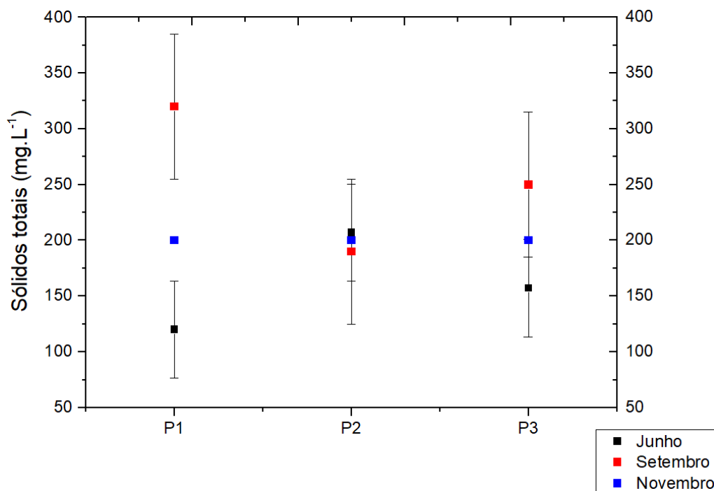
Figura 15 – Variação espacial e sazonal de sólidos totais na água do rio da Prata.
