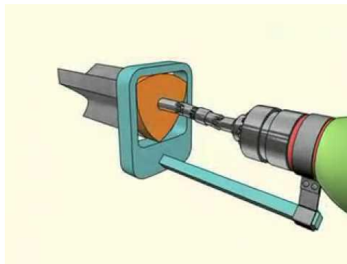
Figura 29 – Furadeira com eixo móvel Disponível em: http://www.youtube.com/watch?v=reKmsqTMwU8 Acesso em: março de 2014
