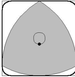
Figura 24 – Trajetória descrita pelo centro do Triângulo de Reuleaux Disponível em: http://beogris.wordpress.com/2007/05/ Acesso em: março de 2014
