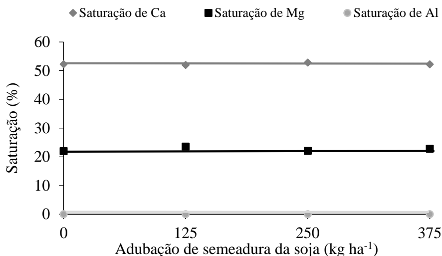
FIGURA 5. Saturação média de cálcio, magnésio e alumínio (%) na profundidade 0-0,2 m em função dos níveis de adubação de sementeira da soja em sucessão ao milho segunda safra.
