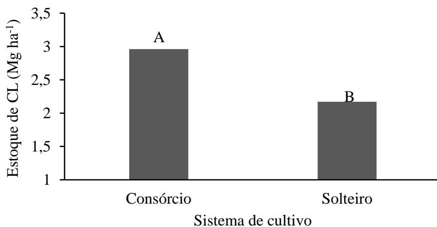
FIGURA 8. Estoque de carbono lábil (CL) em Mg ha -1 na profundidade 0-0,2 m em função dos diferentes sistemas de cultivo do milho segunda safra (solteiro ou consorciado com B. ruziziensis ).
