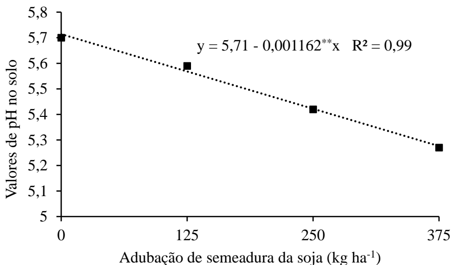
FIGURA 2. Valores de pH CaCl 2 no solo na profundidade 0-0,2 m em função dos níveis de adubação de semeadura da soja em sucessão ao milho segunda safra.
