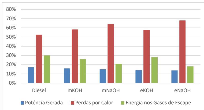
Figura 3 - Distribuição da energia do combustível no sistema
