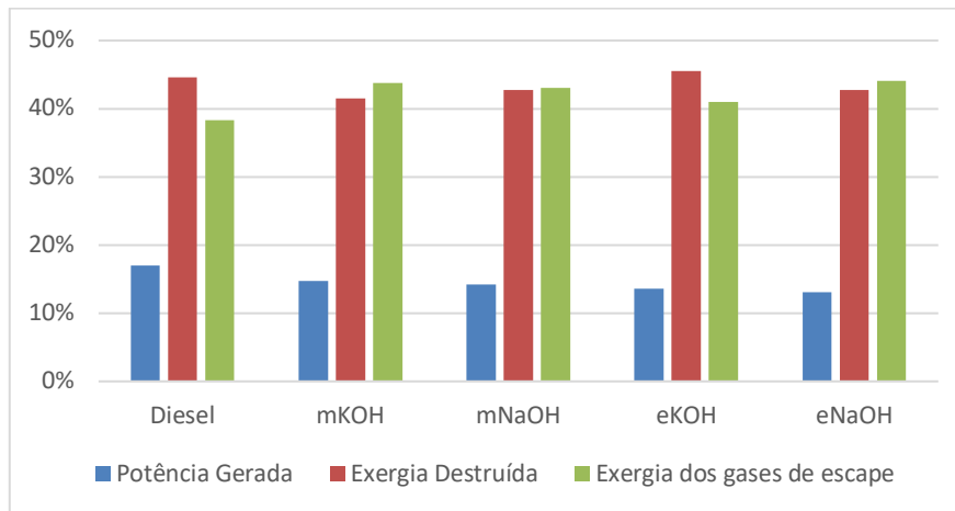
Figura 4 - Distribuição da exergia do combustível no sistema
