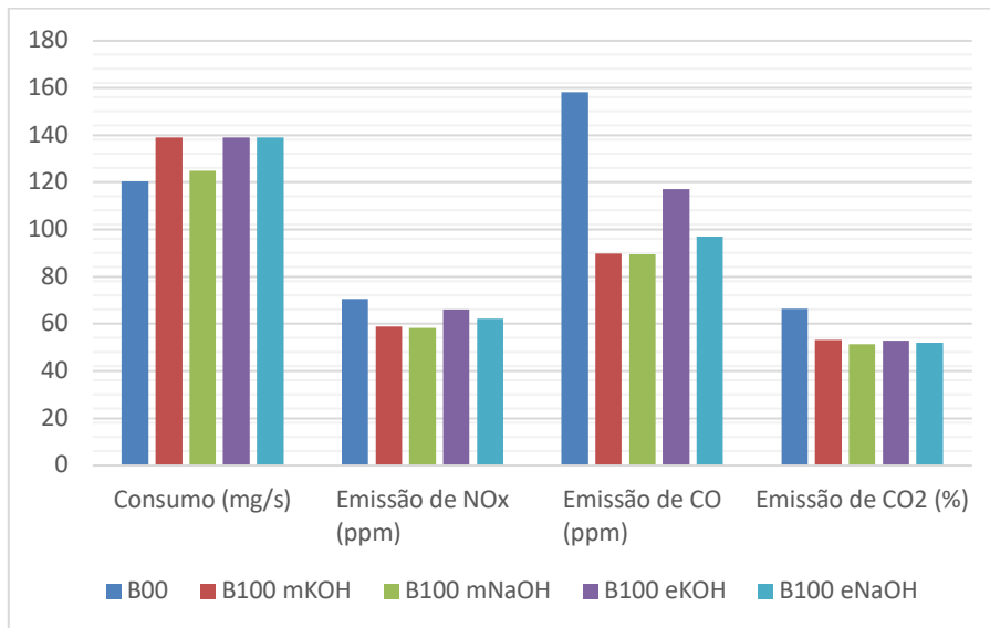
Figura 2 – Comparativo de consumo e emissão de poluentes das amostras B100 e B00
