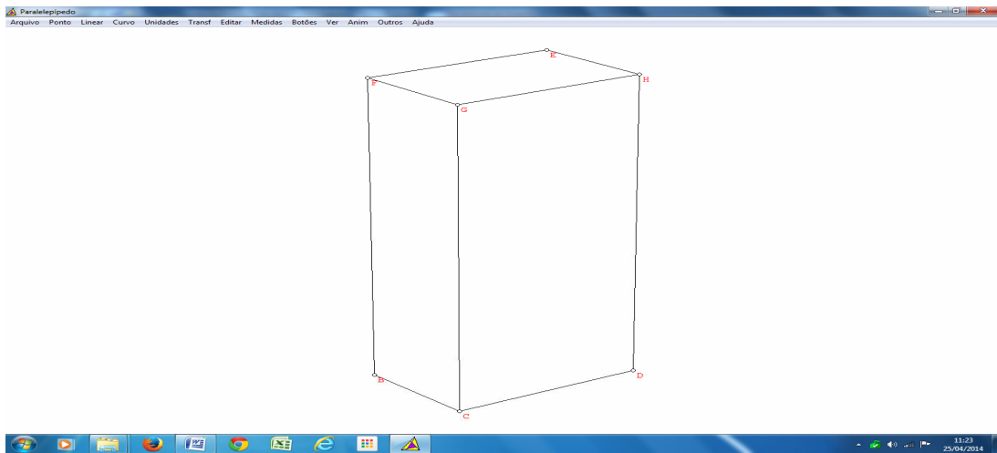
Figura 1:Paralelepípedo
